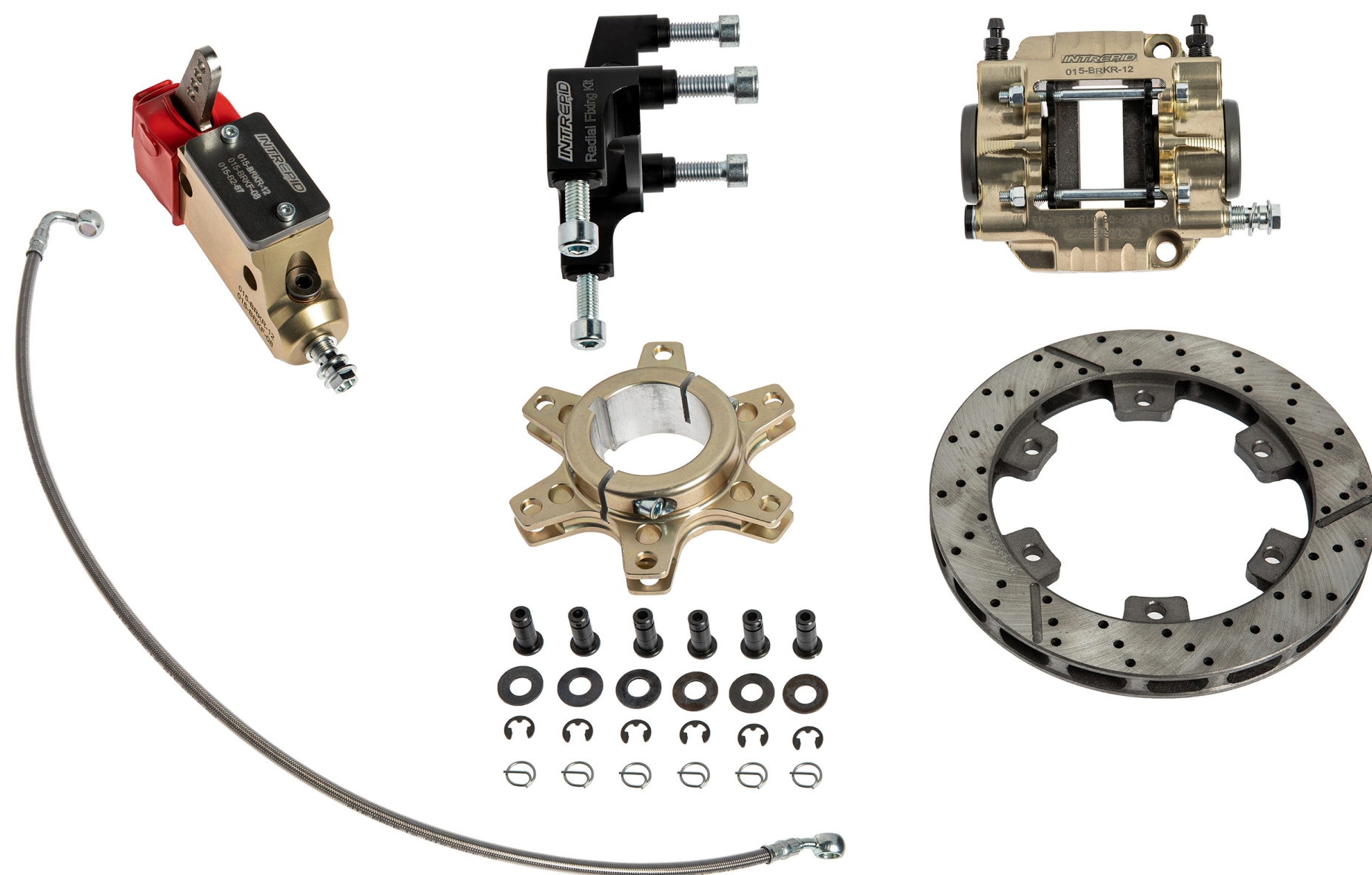
IMPIANTO FRENO
